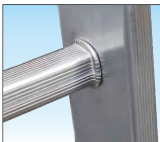
Piolo quadro mm. 30 x 30 anti-scivolo molto robusto con doppia bordatura Unione tra piolo e montante con doppia bordatura, interna ed esterna, per la massima solidità contro urti accidentali ed una lunga durata nel tempo
